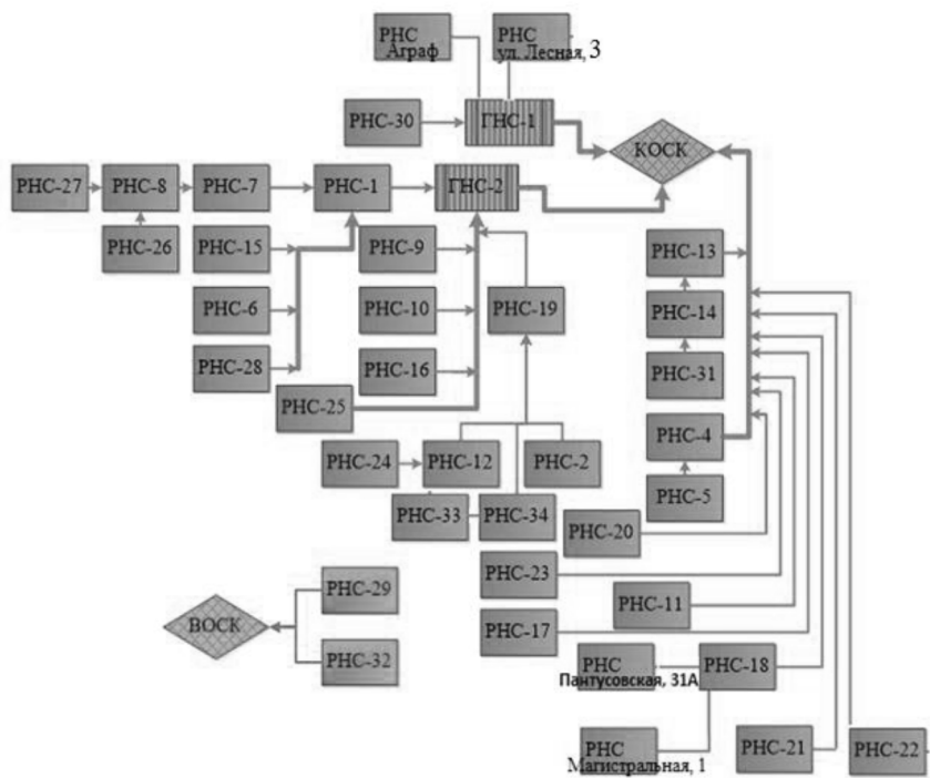
Рисунок 3-13. Структура централизованного водоотведения г. Кострома
