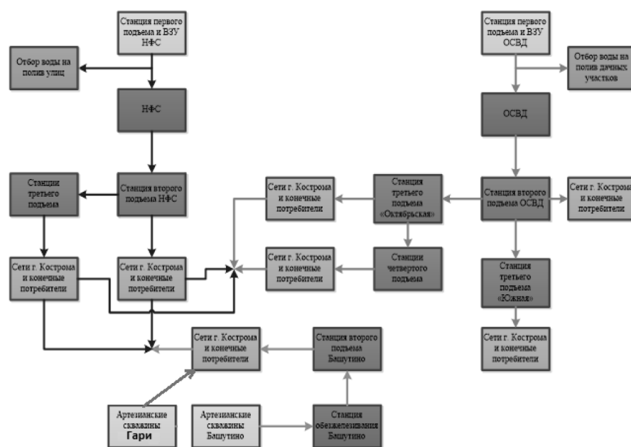
Рисунок 3-9. Структура централизованного водоснабжения города.
