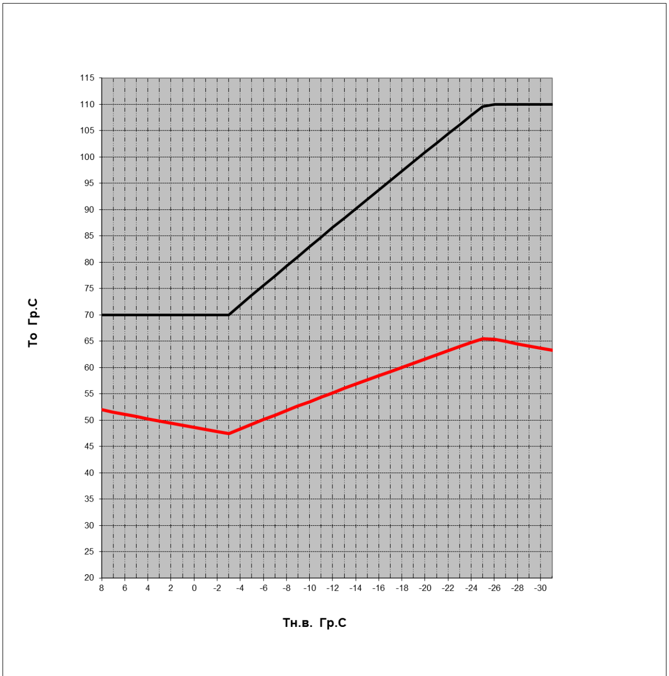
График 4.8.5
