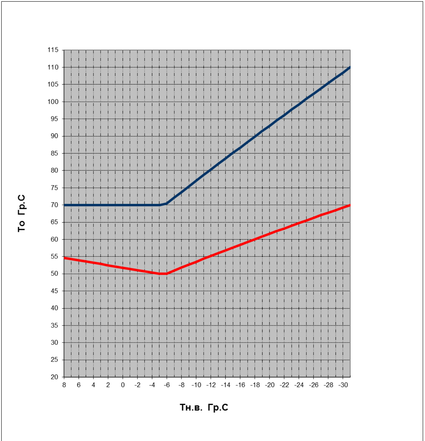
График 4.8.14
