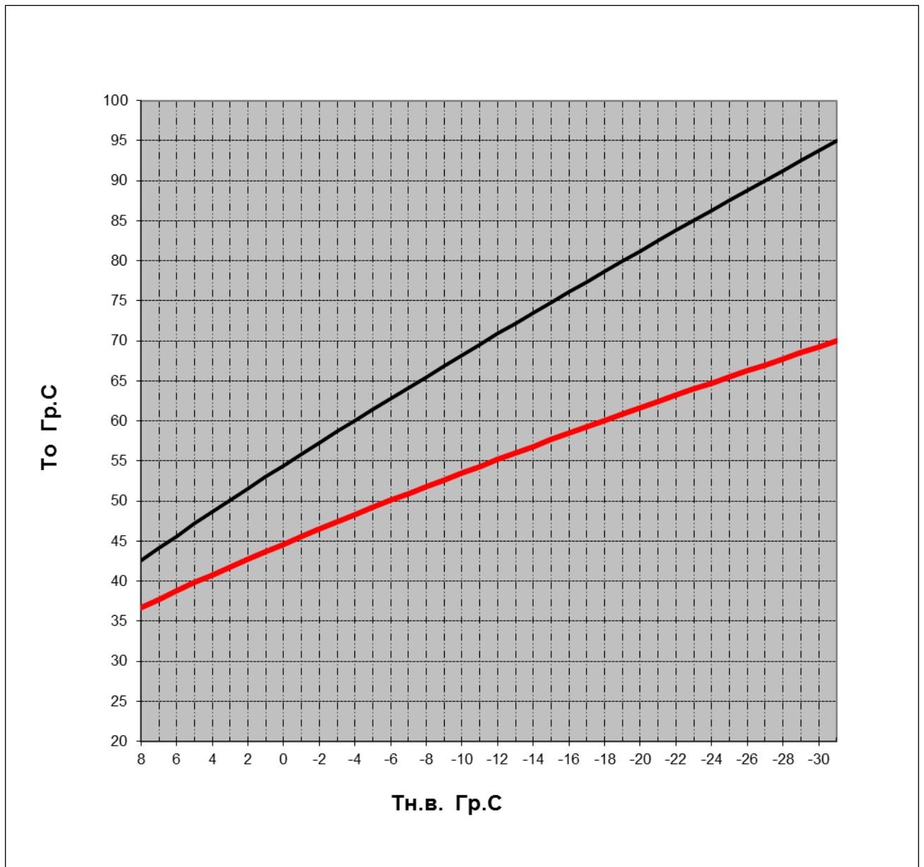
График 4.8.13
