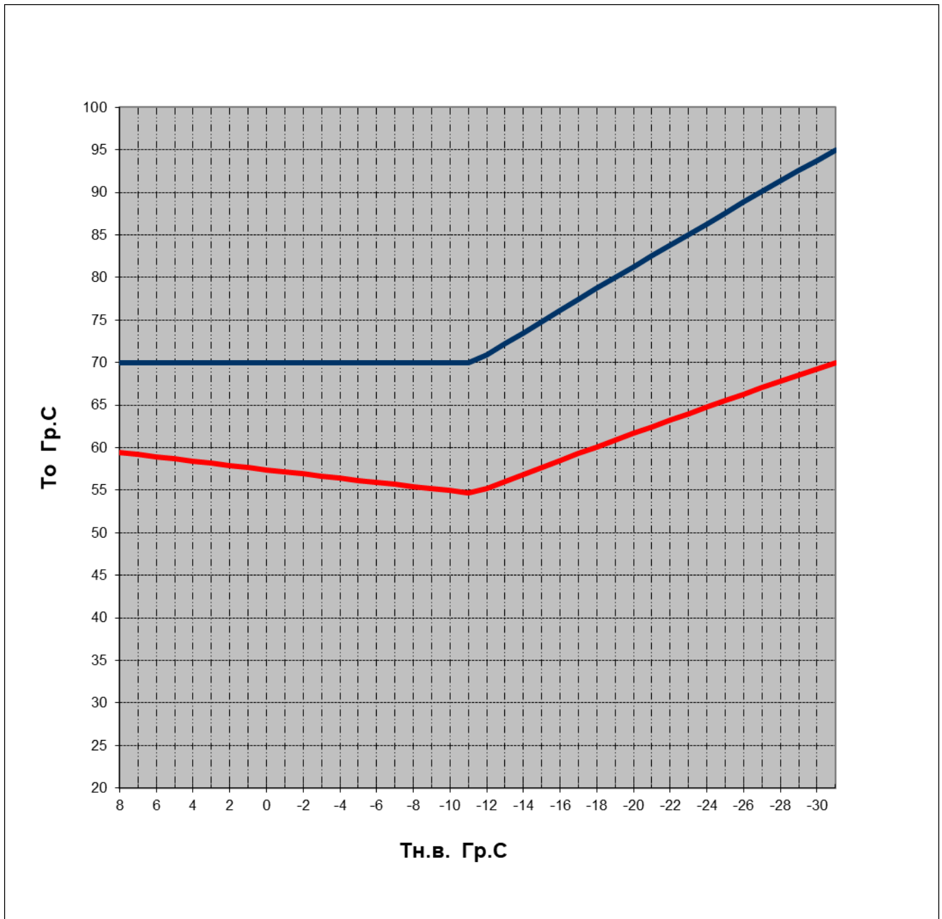
График 4.8.9
