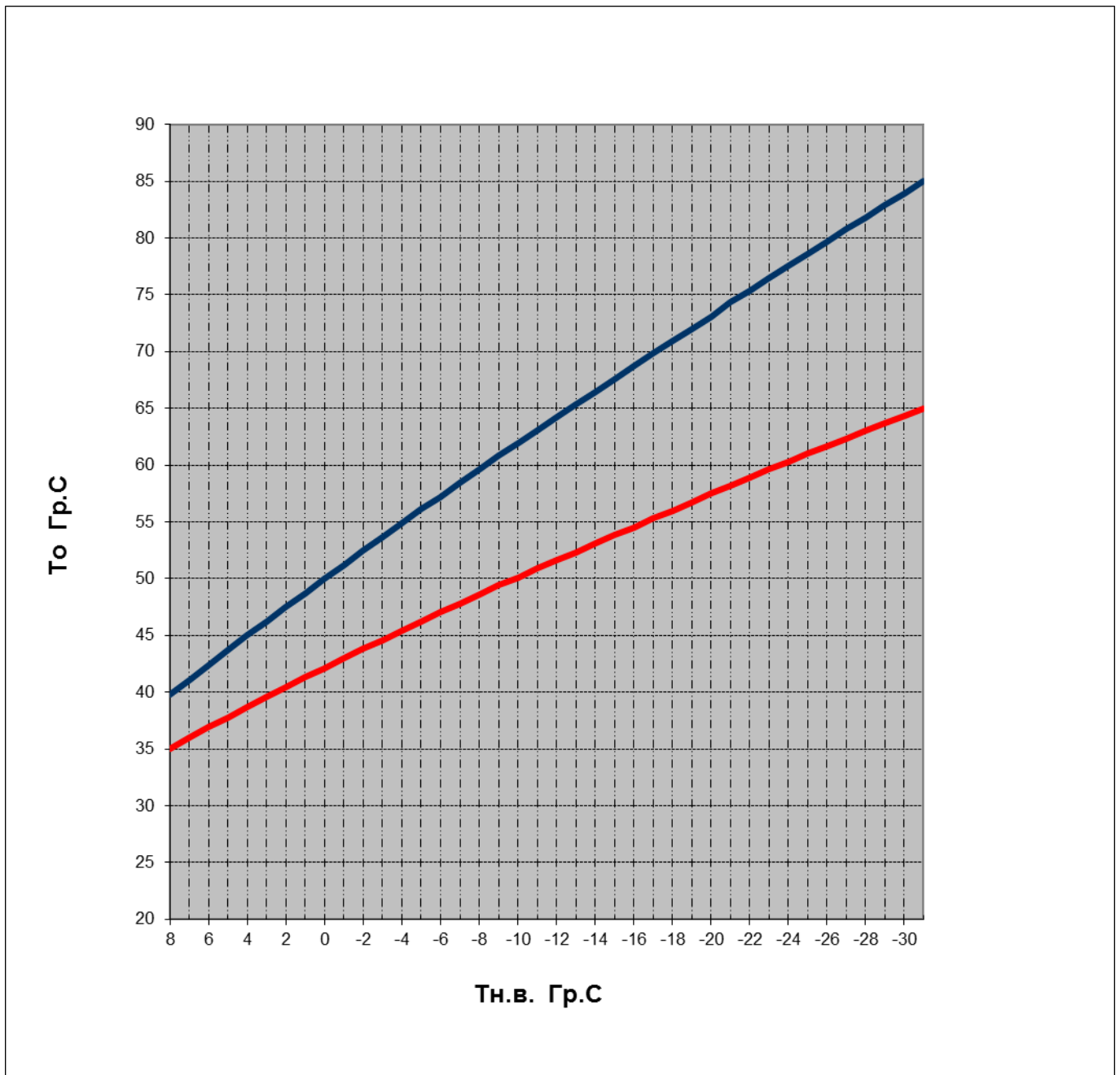
График 4.8.18
