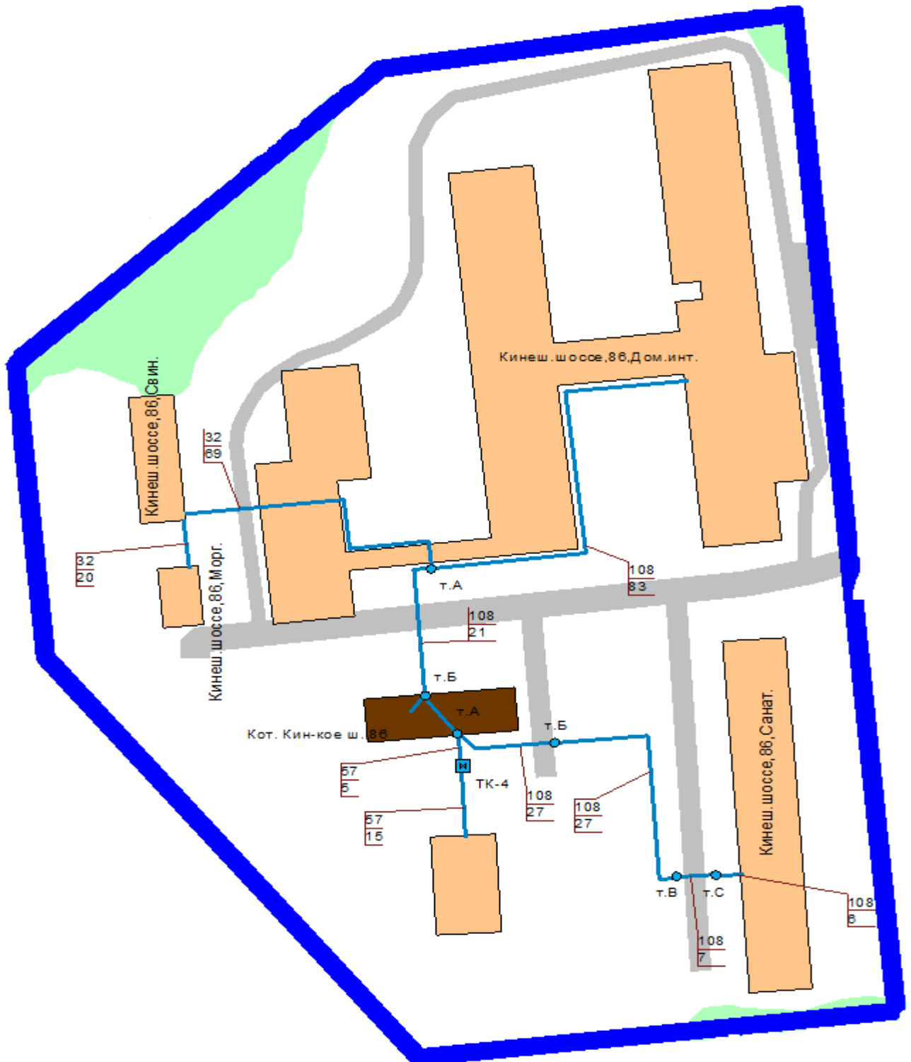
Схема 2.2.17
