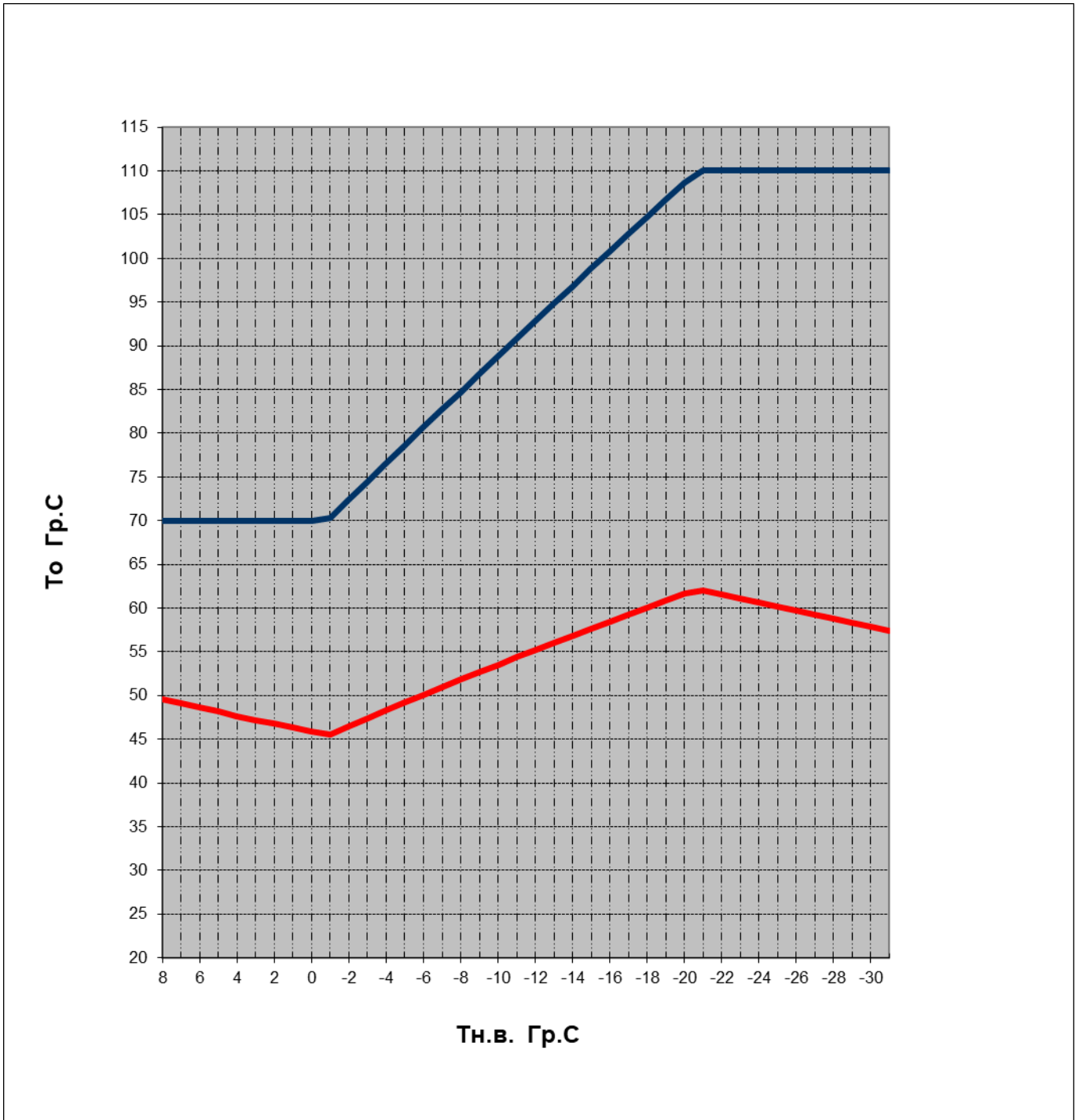
График 4.8.2
