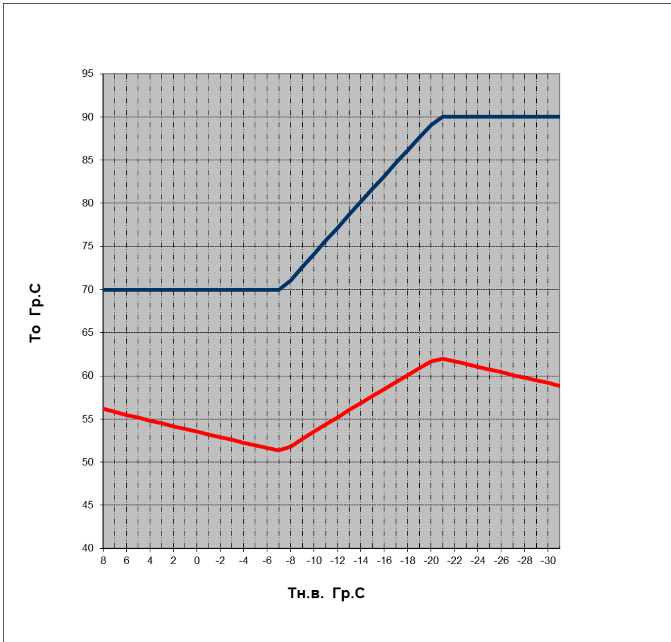
График 4.8.7
